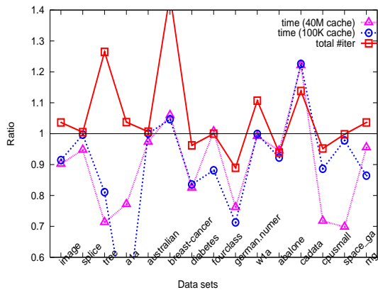
(d) The “final training” step with shrinking
